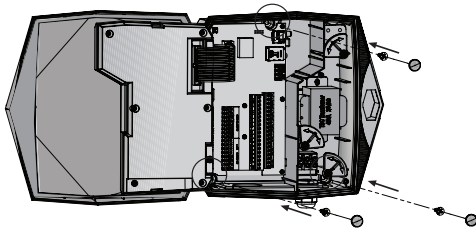
Figura 5: Dimensiones de los tornillos de montaje
