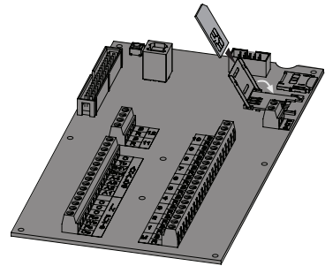
Figura 10: Orientación de inserción de la tarjeta SIM
